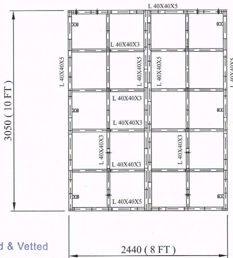
ELEVATION
